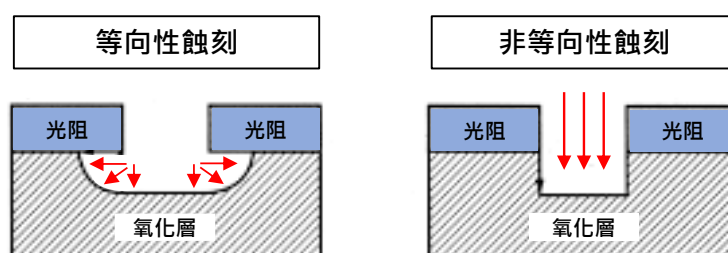
圖 8：非等向蝕刻較等向性蝕刻更能達到先進製程線寬線距需求
